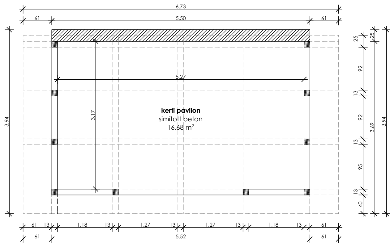
JELENLEGI ÁLLAPOT - ALAPRAJZ - m=1:50
