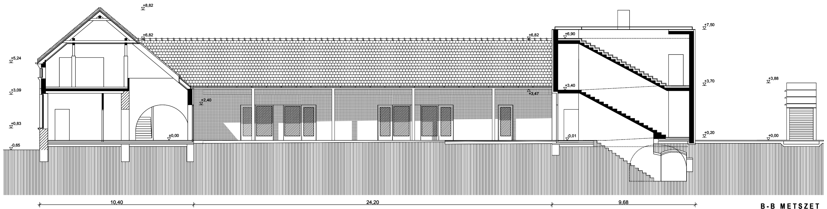
B-B METSZET
