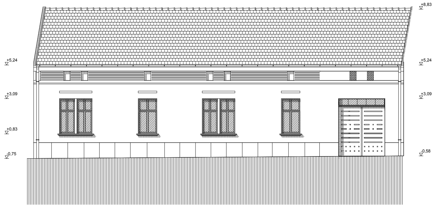
UTCAI HOMLOKZAT
