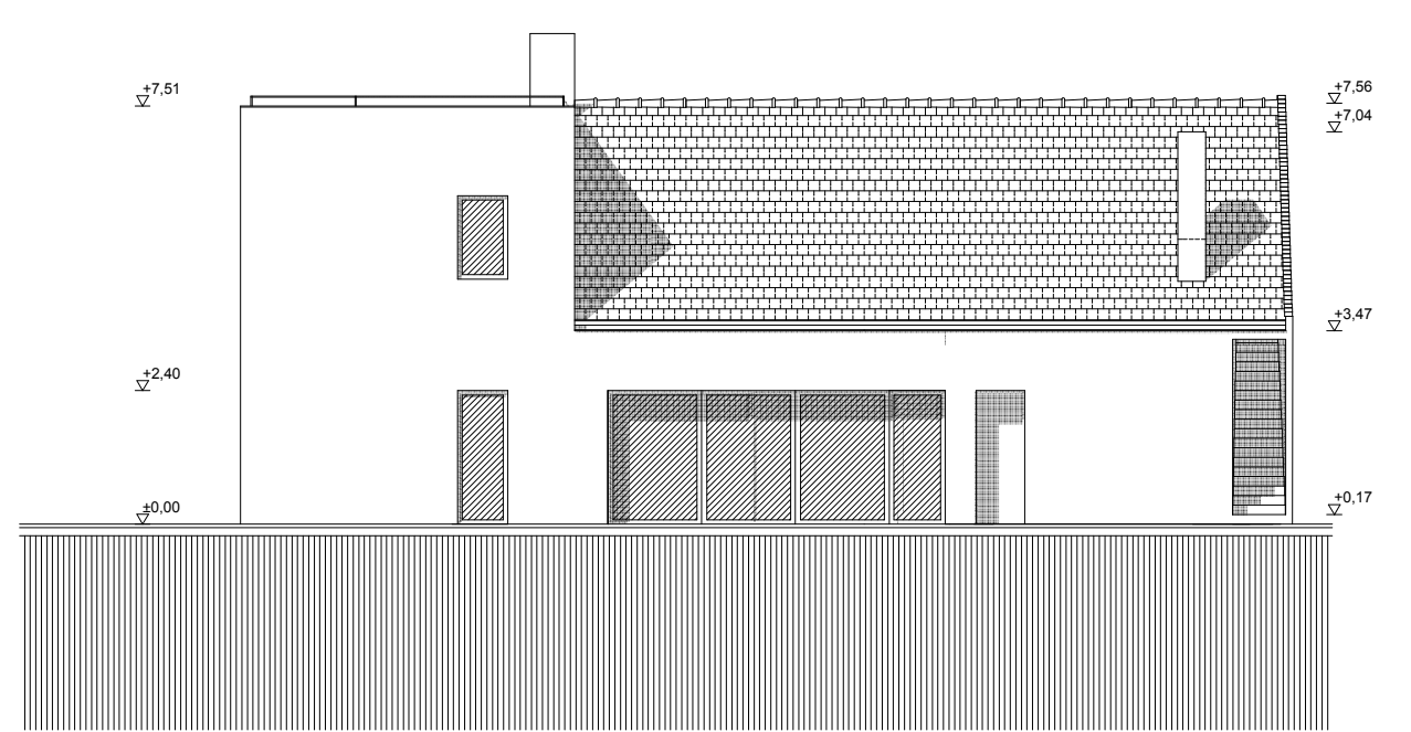
HÁTSÓ HOMLOKZAT
