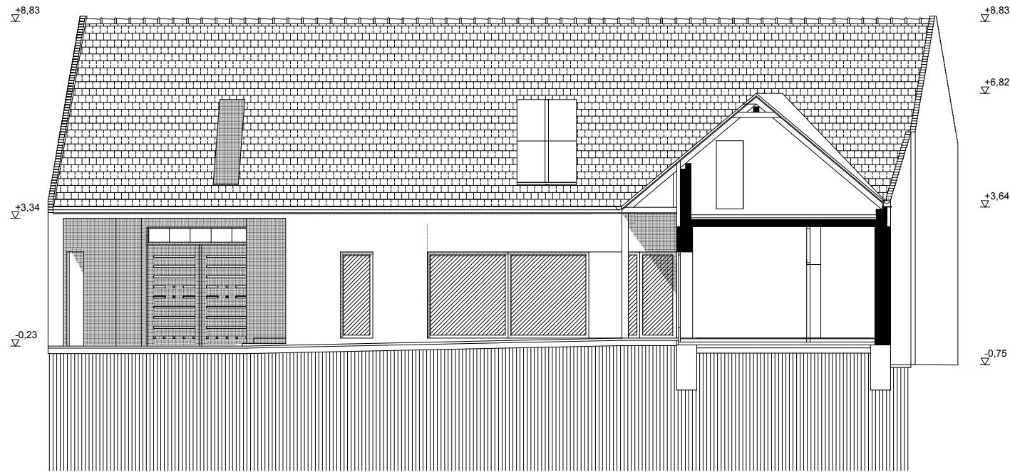
C-C METSZET
