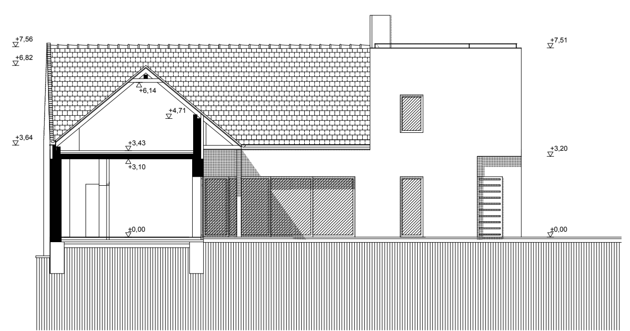
D-D METSZET
