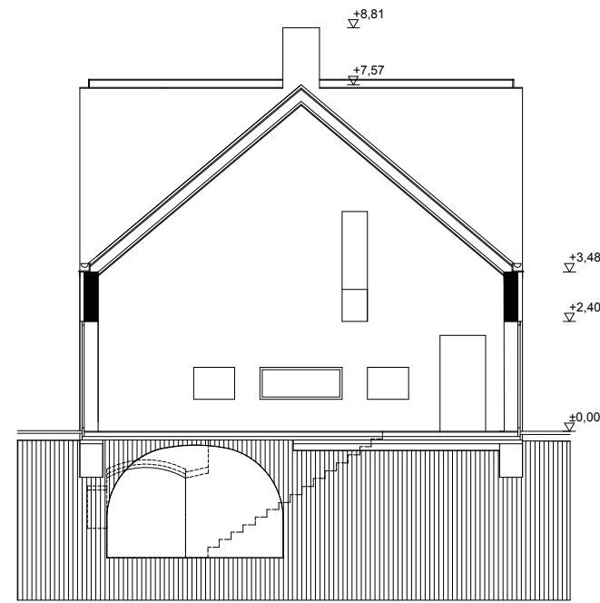
G-G METSZET
