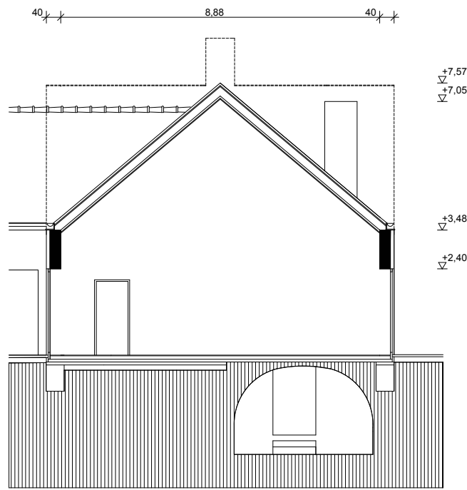
H-H METSZET
