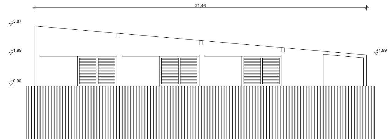
TÁROLÓ HOMLOKZATA
