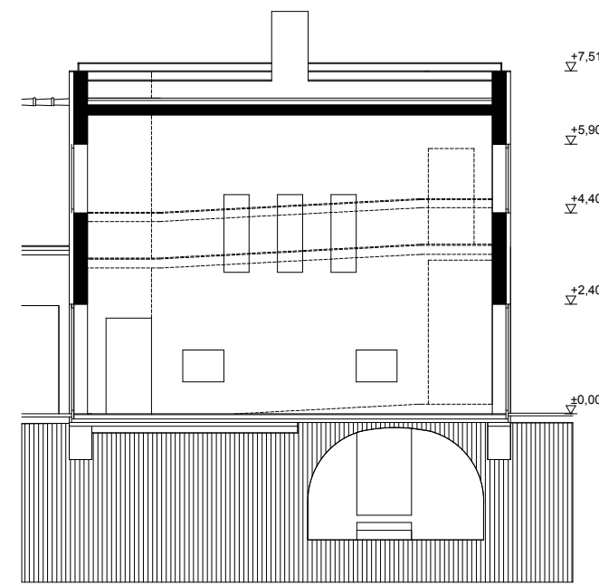
F-F METSZET
