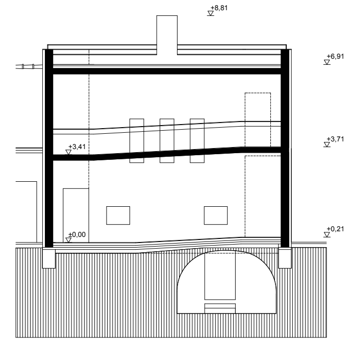
E-E METSZET
