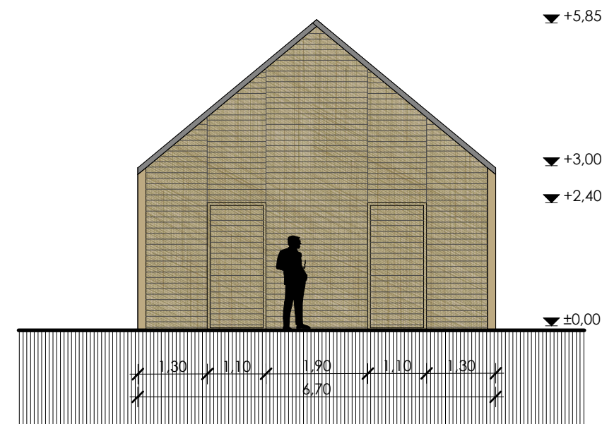
déli homlokzat
