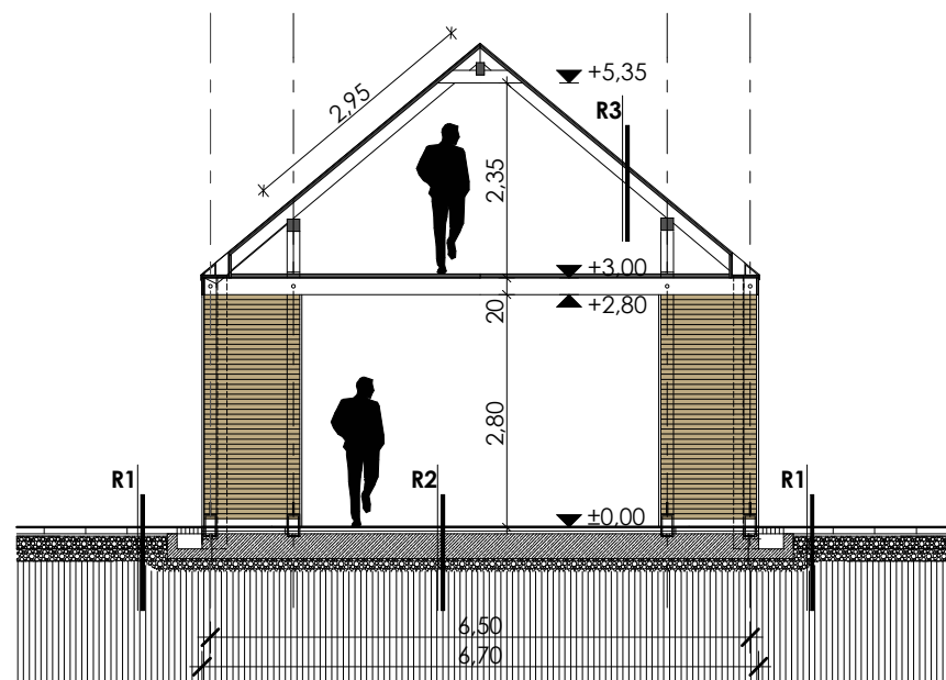
keresztmetszet
